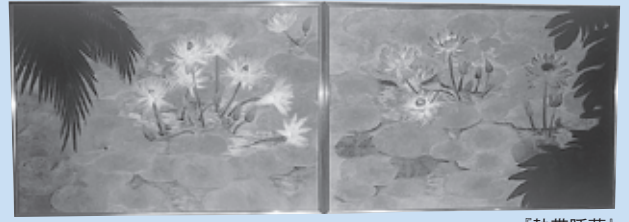
『熱帯睡蓮』
